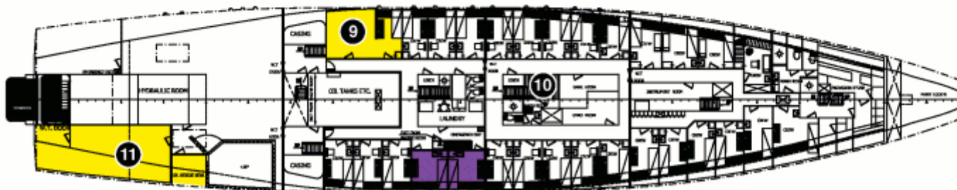
TWEEN DECK 2
